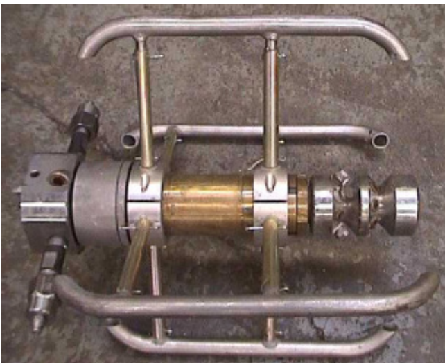
Schlitten mit ca. 200 – 400 mm
